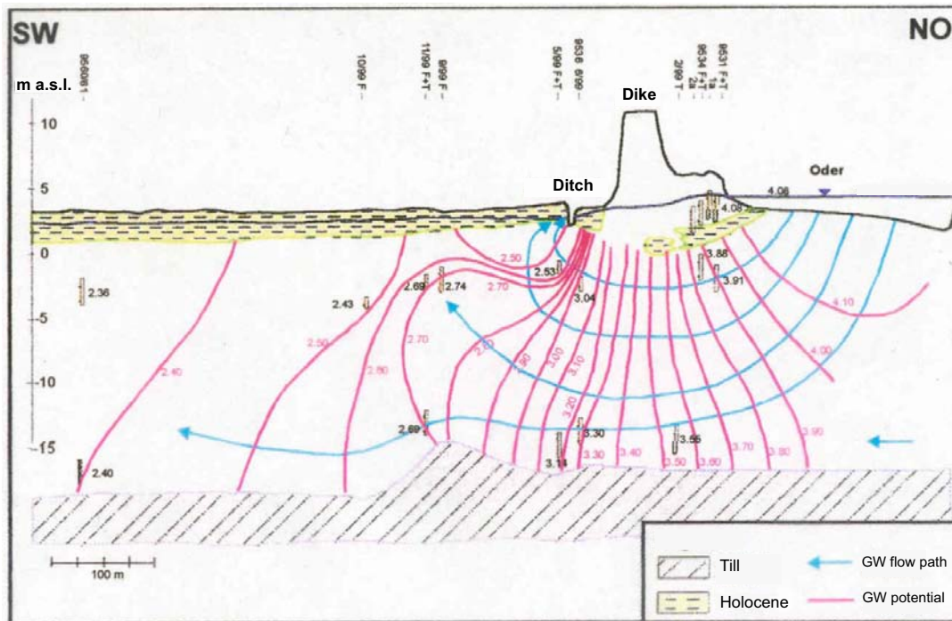
Fig. 4 Seepage under dikes, cross-section of groundwater equipotentials (Massmann 2002) Drängewasserströmung unter Deichen, Äquipotenziallinien (Massmann 2002)
